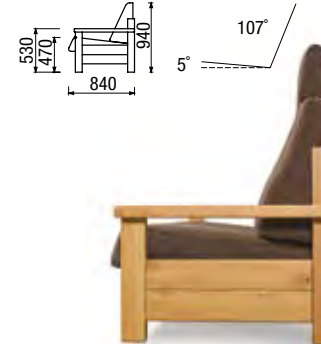
křeslo úložné / rozkládací zvýšené
