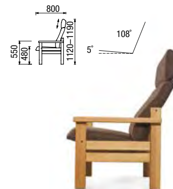
křeslo pevné zvýšené
